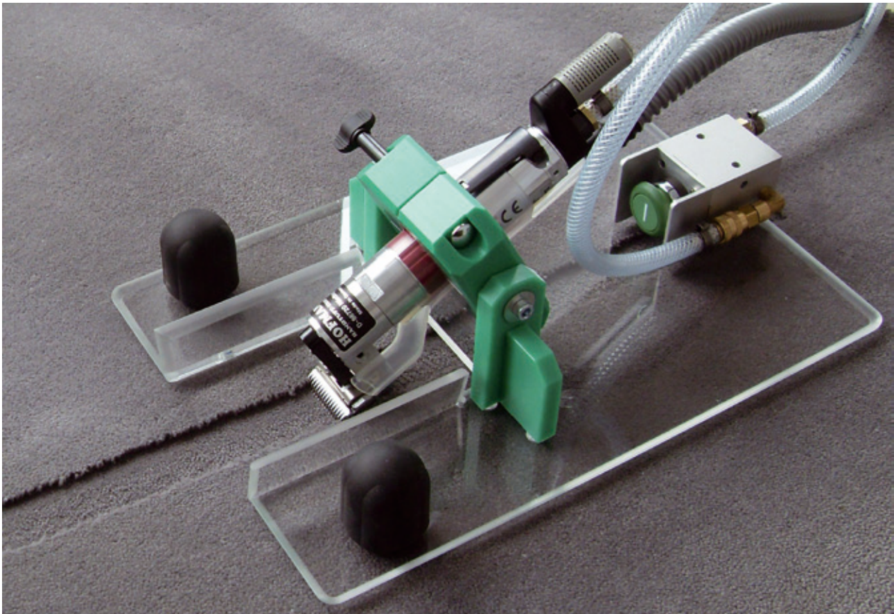
MS 40-A mit Grundplatte / MS 40-A with base plate
