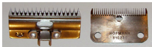
Scherkamm E 895 / Shearing comb E 895
